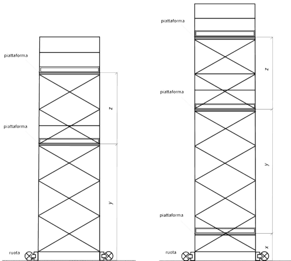
Figura 7.3.1-2: Trabattelli - Altezza dal suolo della piattaforma
