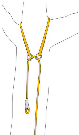
Fig. 8 - Ancoraggio passante per corda raddoppiata
