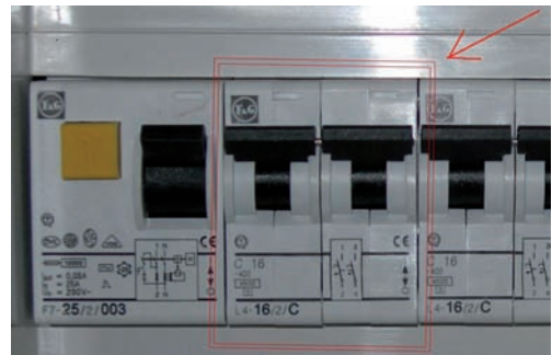
11.18 - Interruttore magnetotermico
