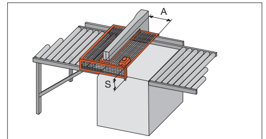
Fig. 10: tunnel su entrambi i lati del piano di taglio. È necessario rispettare le distanze prestabilite per le coperture a tunnel (vedi tabella).
