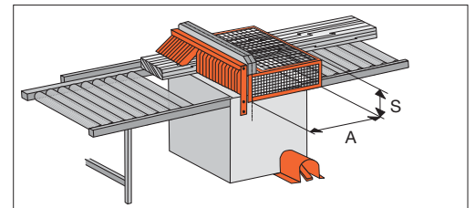
Fig. 9: tunnel con serie di lamelle. In questo modo potete lavorare pezzi di piccole dimensioni. È necessario rispettare le distanze prestabilite per le coperture a tunnel (vedi tabella).
