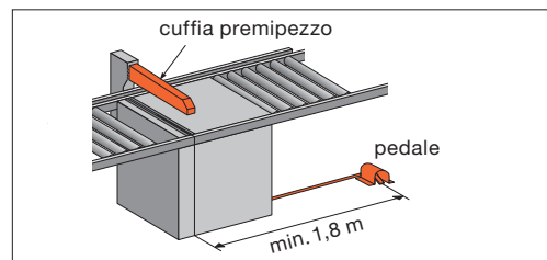
Fig. 7: il pedale è fisso e si trova a 1,8m dalla zona di pericolo. Pertanto, durante la fase di taglio l'operatore non può accedere alla zona di pericolo della lama e della cuffia premepezzo.
