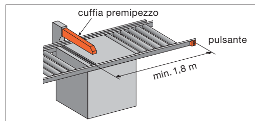
Fig. 6: il pulsante è fisso e si trova a 1,8m dalla zona di pericolo. Pertanto, durante la fase di taglio l'operatore non può accedere alla zona di pericolo della lama e della cuffia premepezzo.
