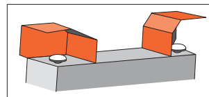
Fig. 2: comando a due mani con copertura
