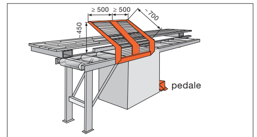
Fig. 8: copertura inclinata. L'estensione del tavolo impedisce che si possa entrare in contatto con la lama dalla parte posteriore.
