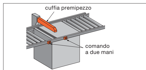
Fig. 5: il comando a due mani impedisce che l'operatore possa entrare con le mani nella zona di pericolo della macchina.
