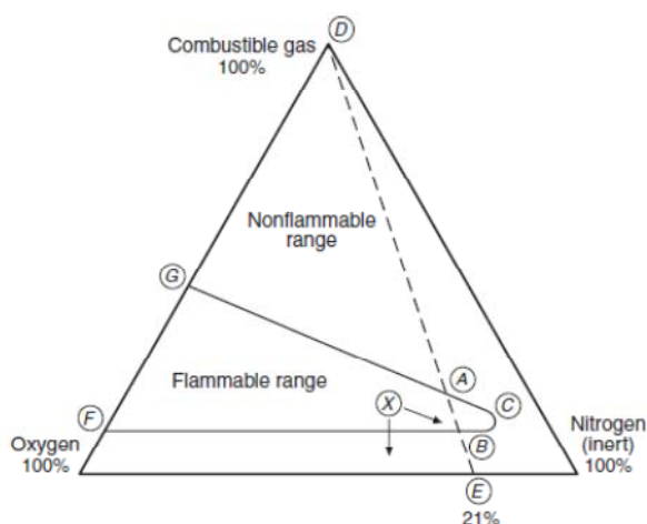
Figura 3 - Diagramma triangolare di esplodibilità relativo ad una generica miscela combustibile-ossigeno-azoto [NFPA 69]
