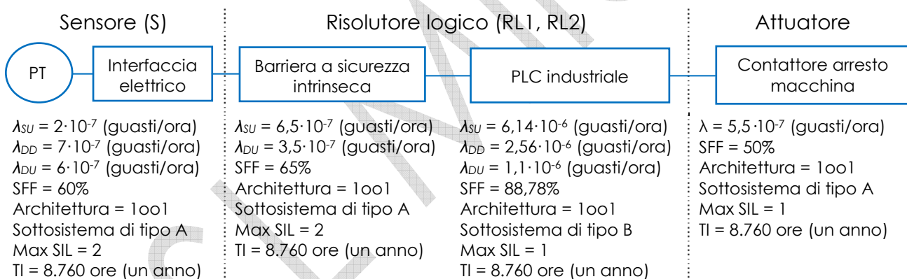
Figura 4.7 – Schema a blocchi – Esercizio - Ipotesi 3
