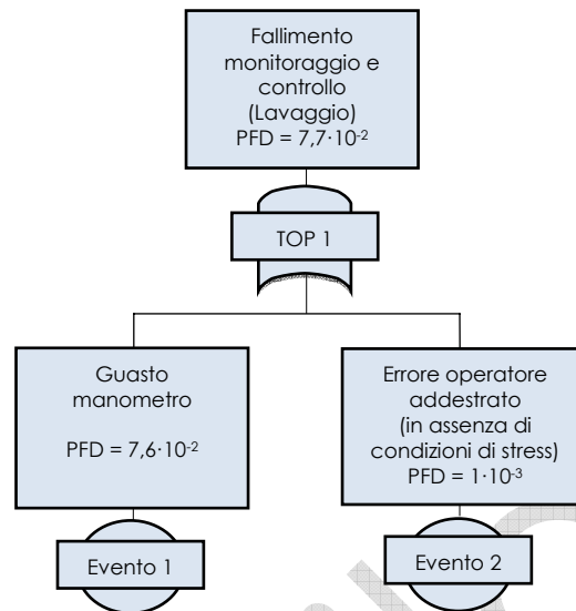
Figura 4.2 - Albero dei guasti - Lavaggio iniziale - Ipotesi 1
