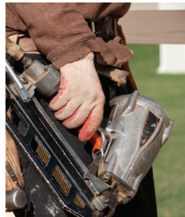
Agarre normal de una pistola de clavos con un dedo en el gatillo
