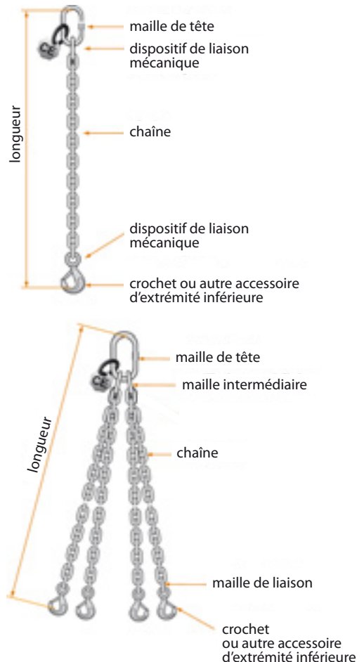
Figure 11 - Élingues chaînes
