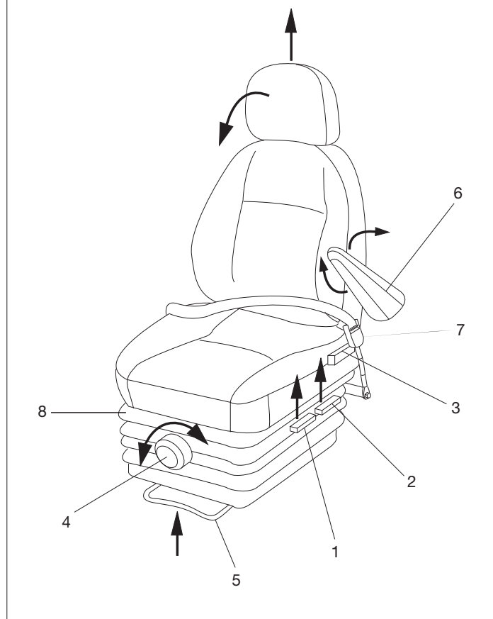
Disegno 5. Esempio di sedile.
