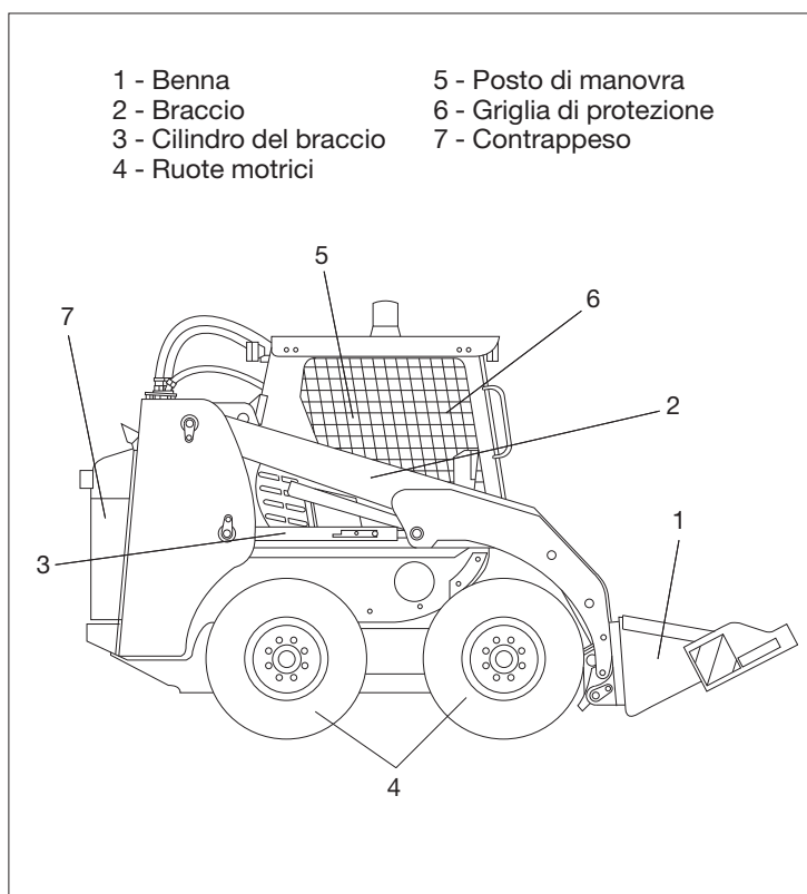
Disegno 3. Pala caricatrice compatta gommata (tratto dalla UNI EN 474-3).
