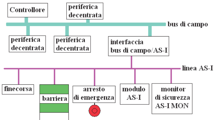
Figura 22: Interconnessione tra dispositivi realizzata con due reti operanti su bus diversi
