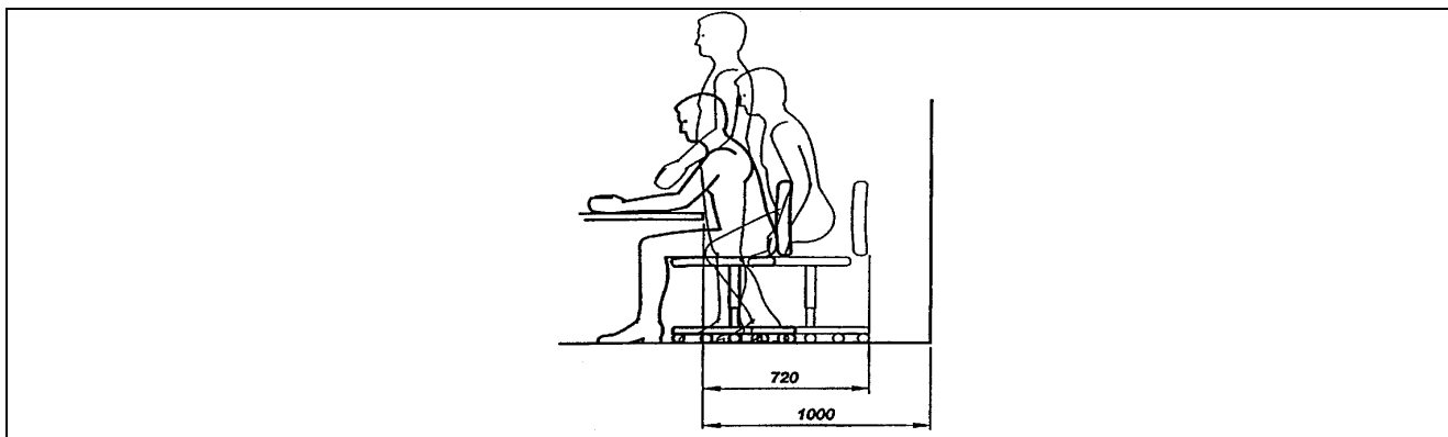
Fig. 3 - figura B.3 UNI EN ISO 14738: progettazione ergonomica – spazio adeguato per il sedile in cassa
