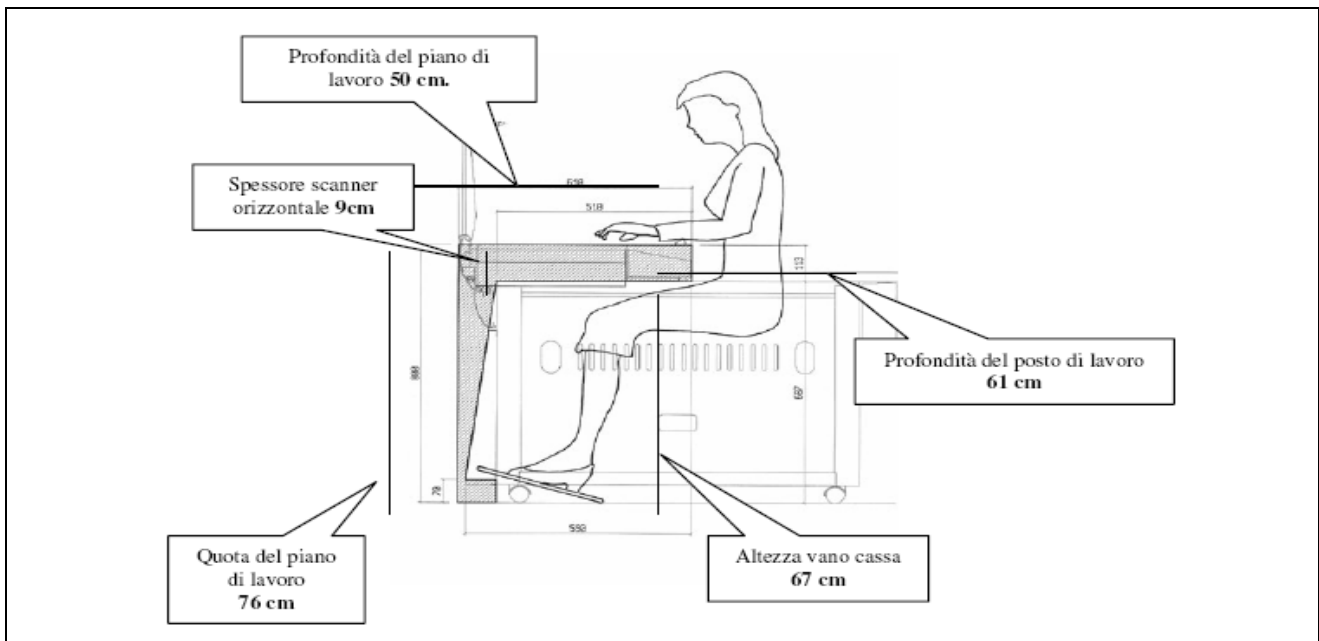
Fig. 4 – L.Guida Reg. Veneto: progettazione ergonomica - parametri dimensionali corretti del posto cassa
