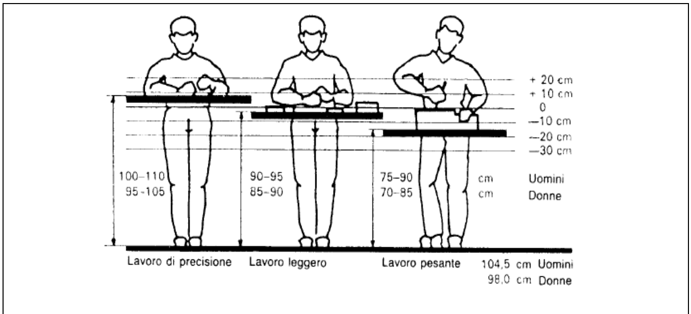
Fig. 35 – altezza adeguata del piano di lavoro in funzione del tipo di attività da svolgere (Codice del Comitato Nazionale Svedese per la salute e la sicurezza del lavoro) che, secondo Grandjean, va riferita all'altezza del gomito.
