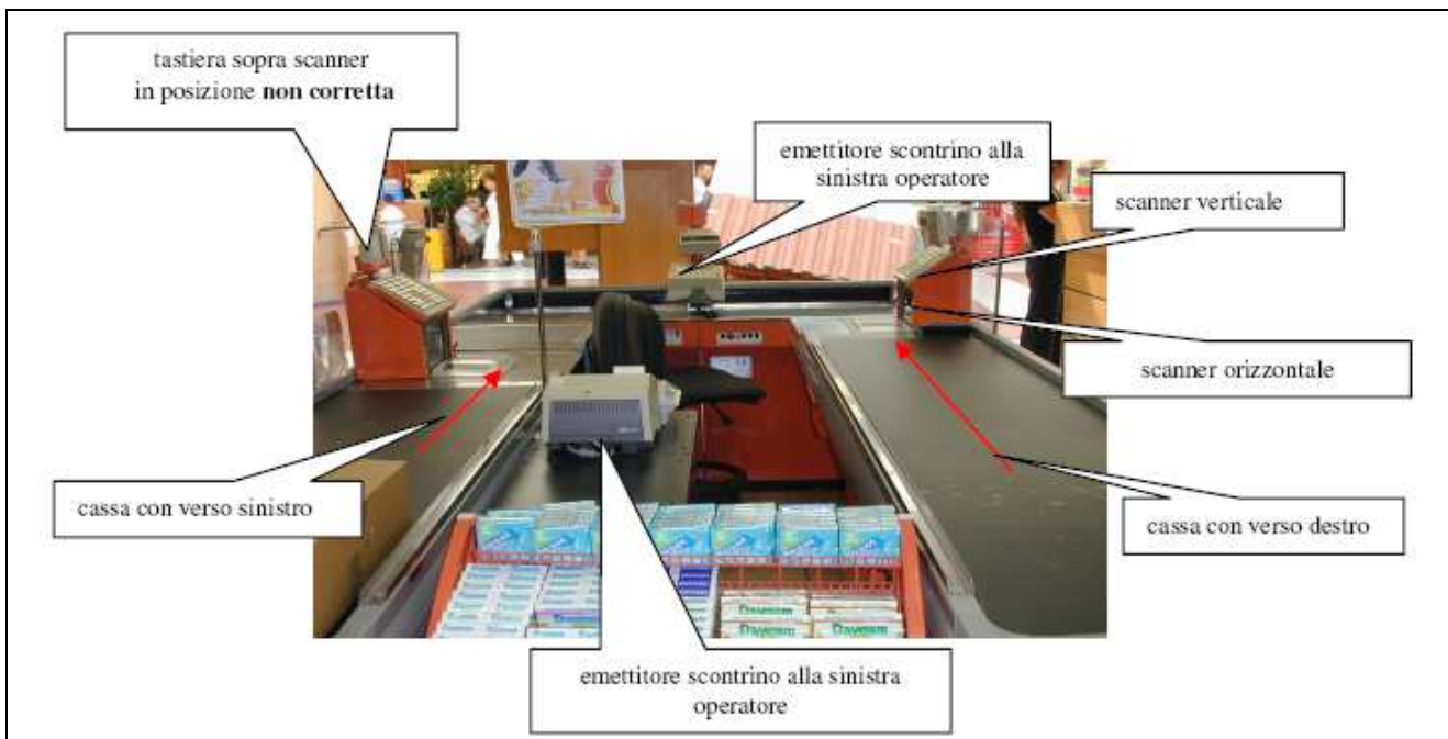
Fig. 2 – L.Guida Reg. Veneto: posto cassa corretto con ingresso merce bidirezionale (cassa a isola)
